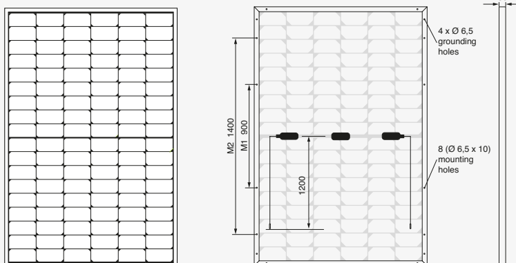
Abb. Prinzipskizze
